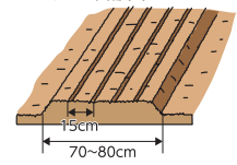
図3 トンネルの被覆
